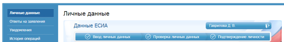
Рисунок 6. Данные ЕСИА.
